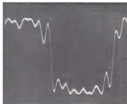
blokgolf van 1002 Hz uit de MD-speler
